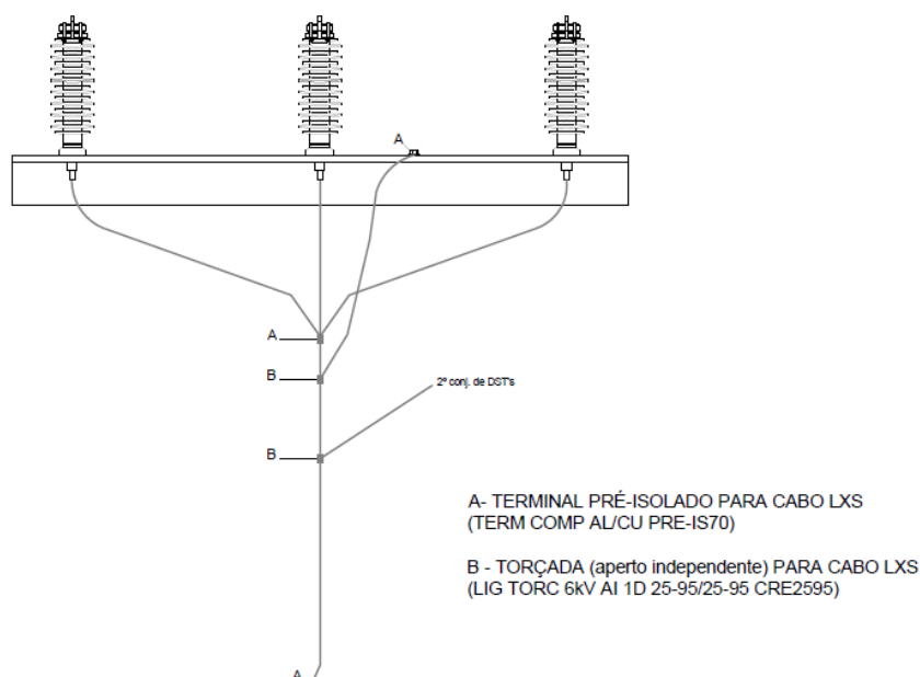
Fig. 6A - Ligação à terra dos DST
