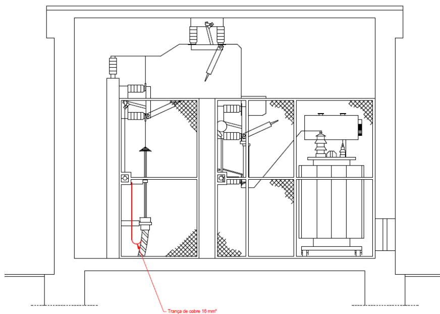
Fig. 13 – LSMT • Ligação das bainhas dos cabos à terra
