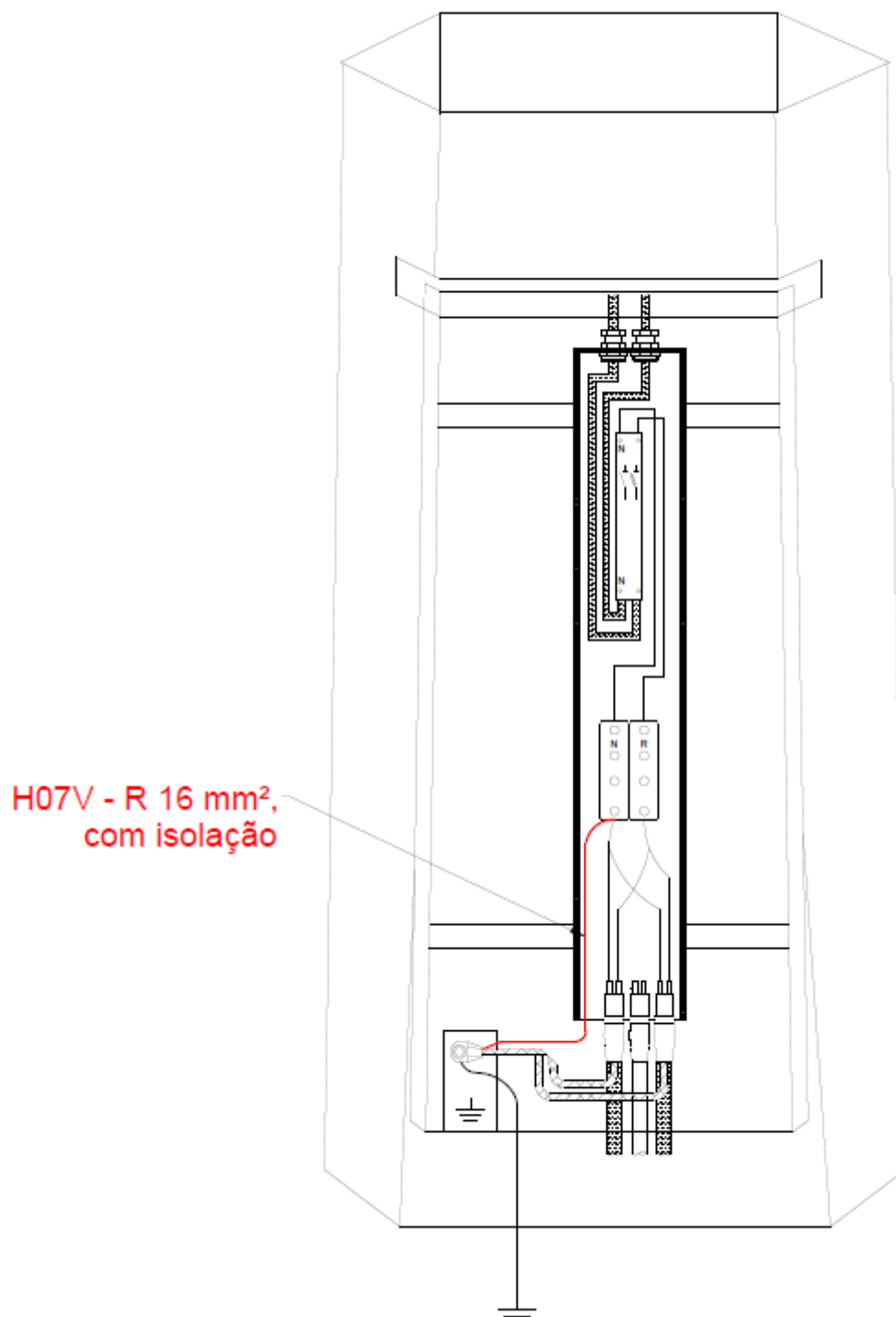
Fig. 2F – RSIP • Ligação do borne de neutro do Quadro IP ao terminal do fuste da coluna
