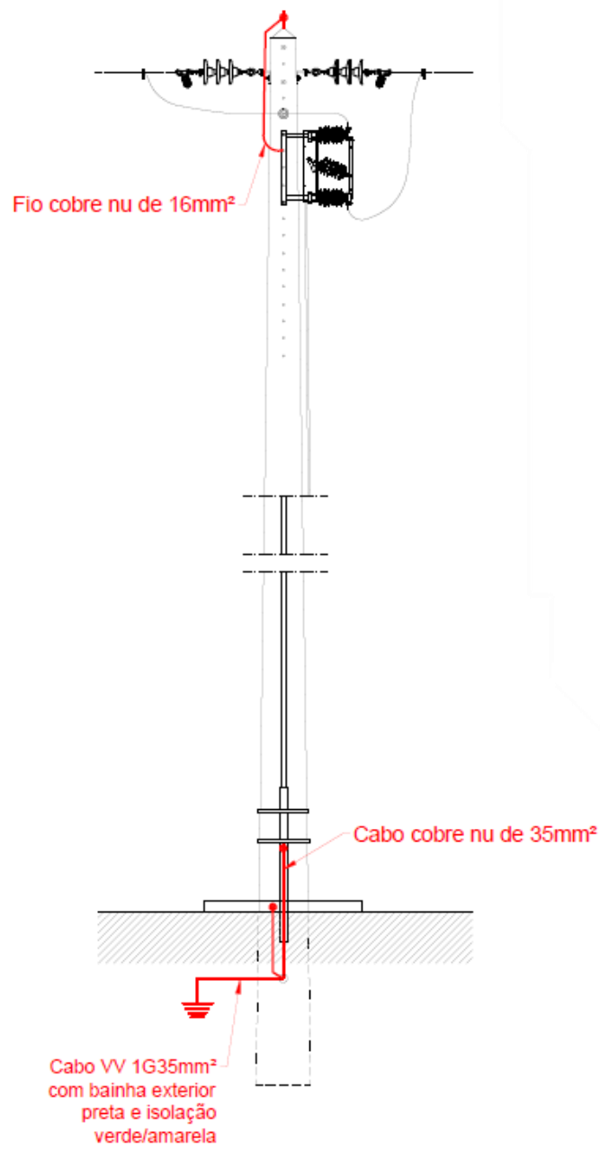
Fig. 5 – LAMT – Ligações à terra em poste com seccionador
