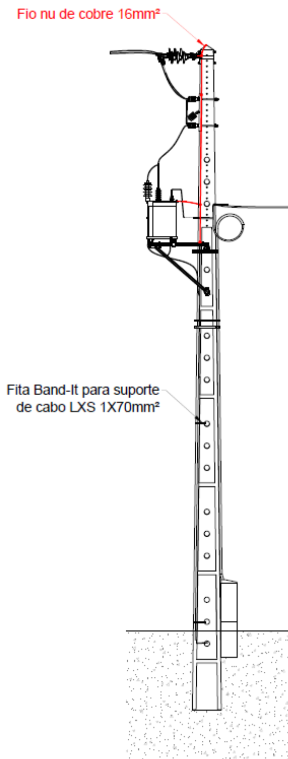
Fig. 10B – PT aéreo tipo R250 e AI • Ligação da armação de suporte e tampa do TP + interruptor-seccionador + HPT4, à terra
