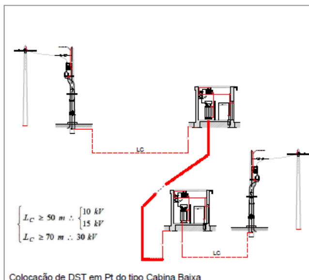
Fig. 23 - PT do tipo CB • Ligação de DST
