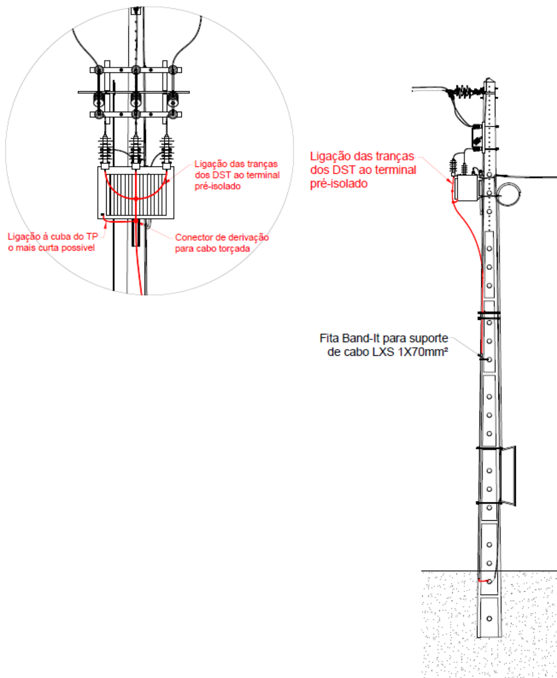
Fig. 16 - PT aéreo tipo R100•Ligação DST à terra
