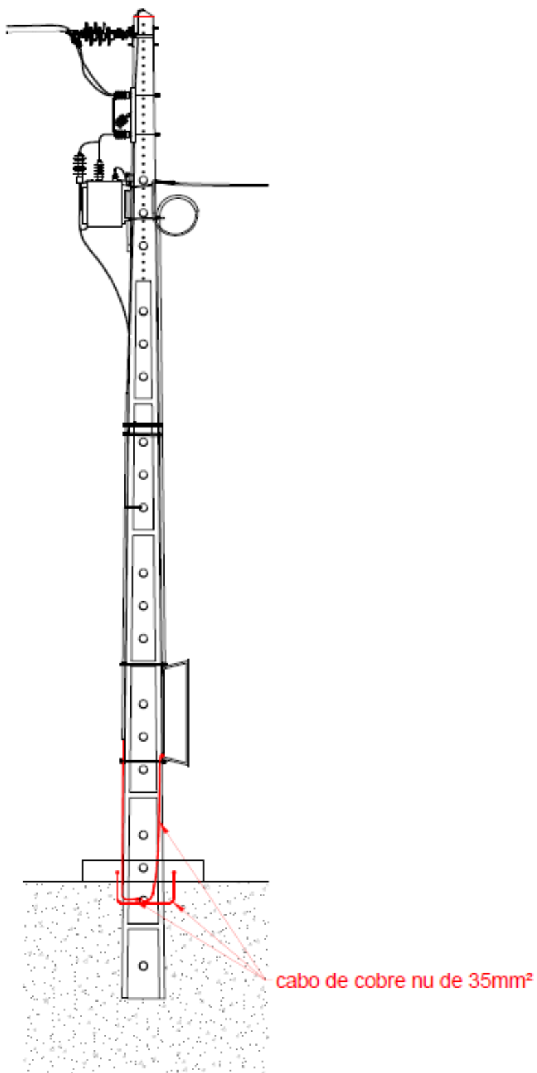
Fig. 7B – PT aéreo tipo R100 e AS • Ligação das plataformas + comando do seccionador + QGBT, à terra
