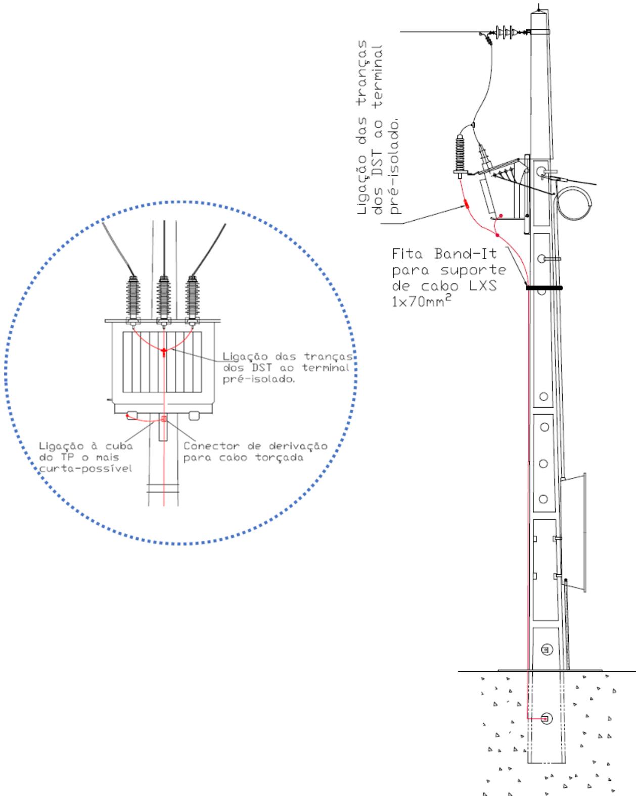
Fig. 1B – PT aéreo tipo A • Ligação dos DST à terra e à cuba do TP
