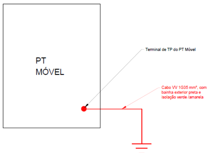
Fig. 11.3 – PT Móvel • Ligação aos eletrodos de terra
