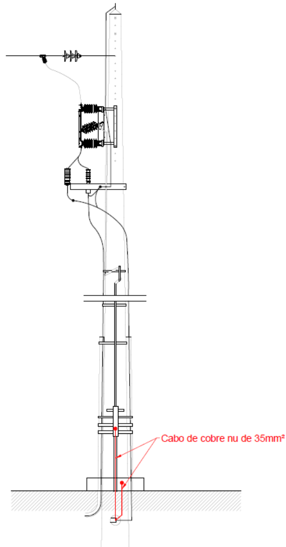
Fig. 9 – LAMT/LSMT • Ligação plataformas + comando do seccionador à terra
