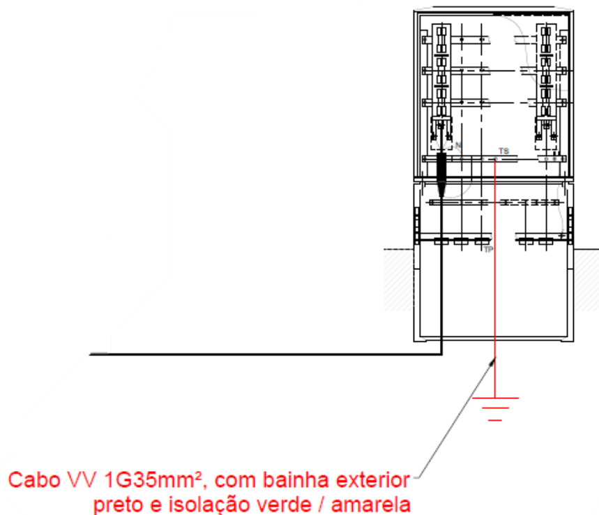
Fig. 29 - RSBT • Ligação neutro à terra (caso geral)
