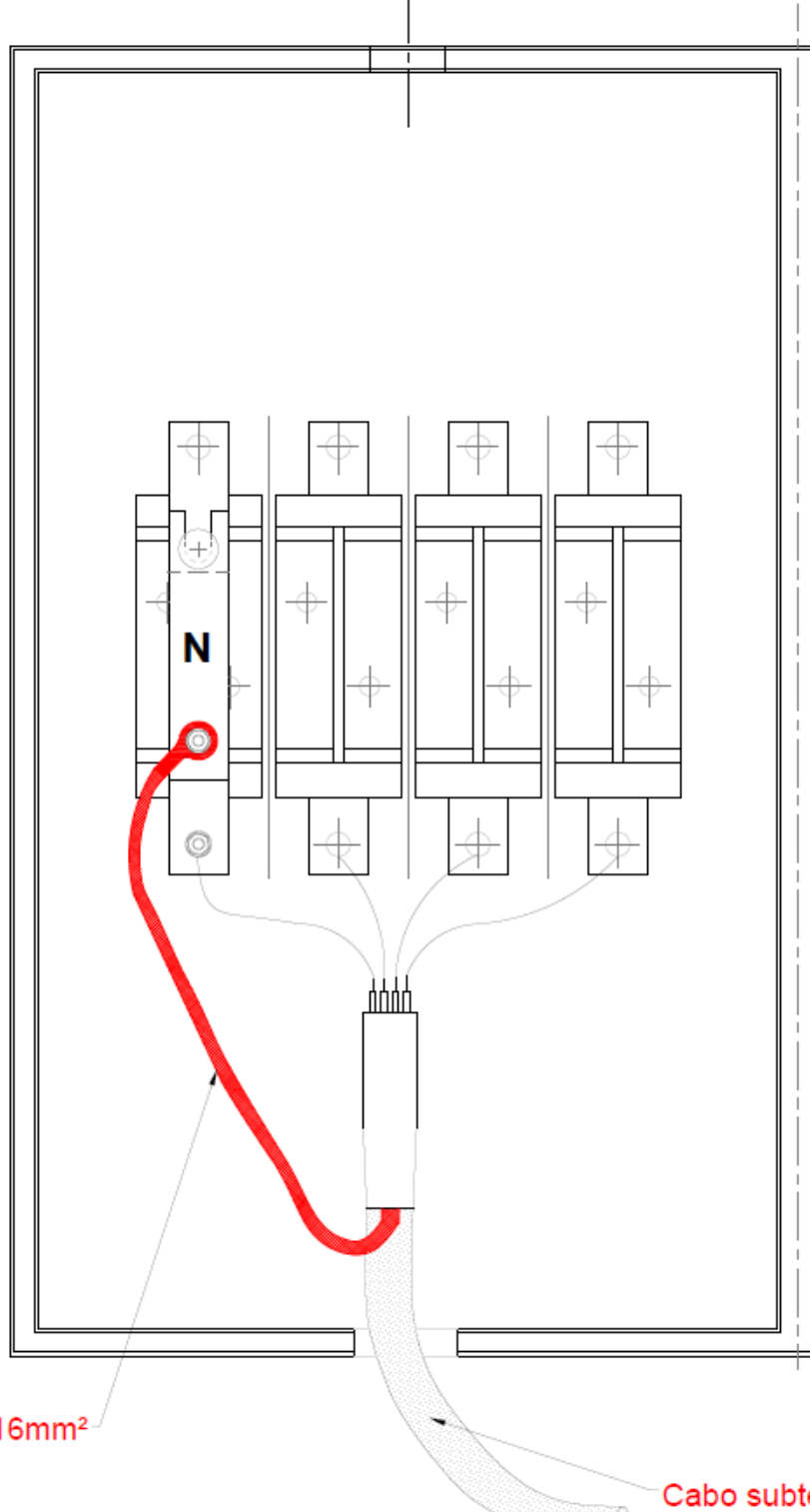
Fig. 1E – Ramais BT • Ligação das terminações dos cabos subterrâneos ao barramento de neutro
