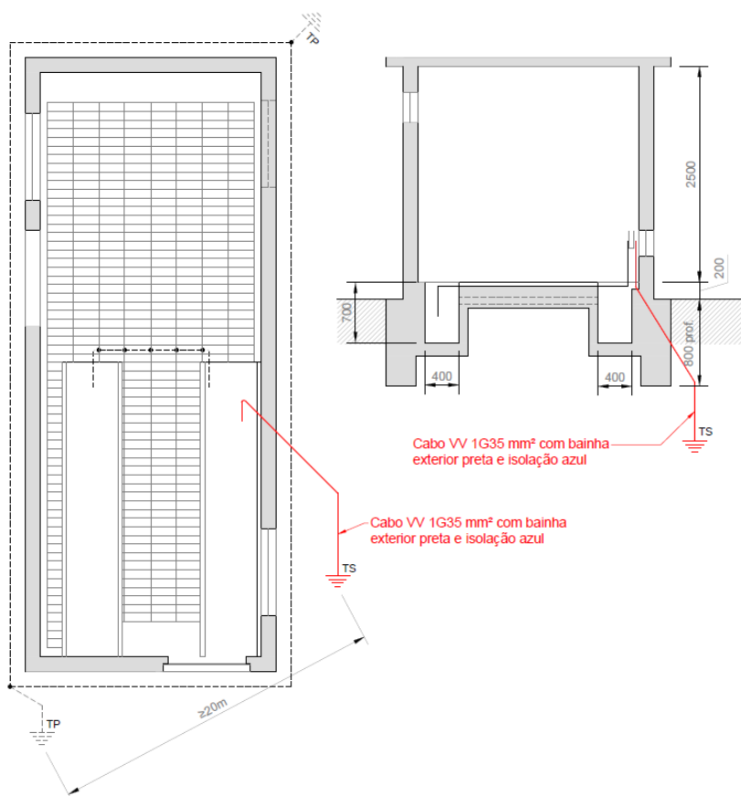
Fig. 27 – PT tipo CB • Ligação do neutro à terra de serviço
