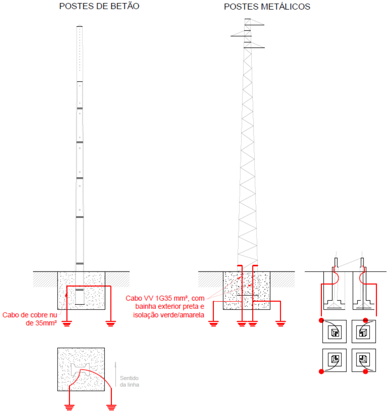
Fig. 1A – LAMT Ligação do terminal de terra inferior dos postes aos elétrodos de terra
