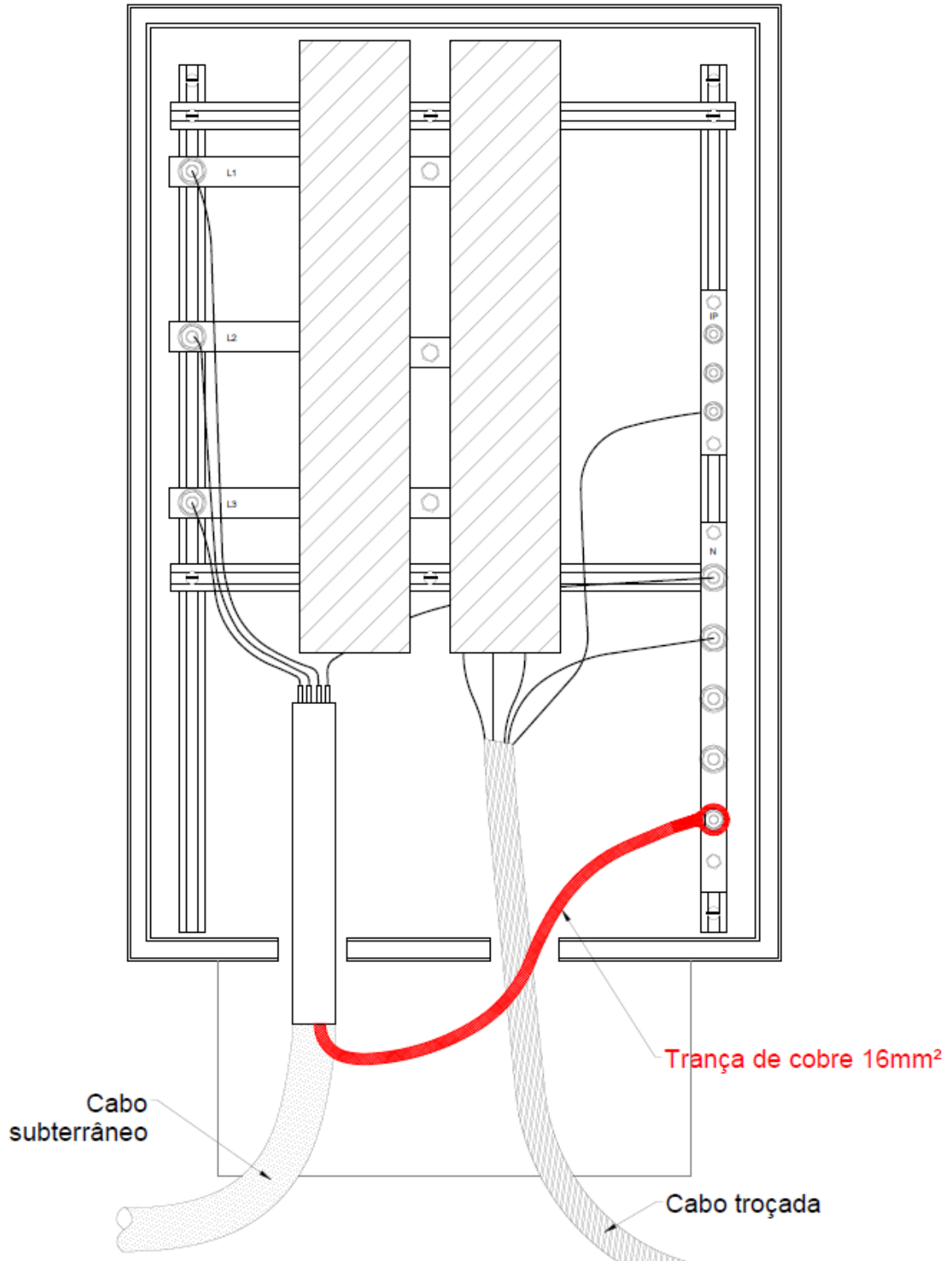
Fig. 4D – RSBT/RABT • Ligação das terminações à terra em transições aéreo-subterrâneas
