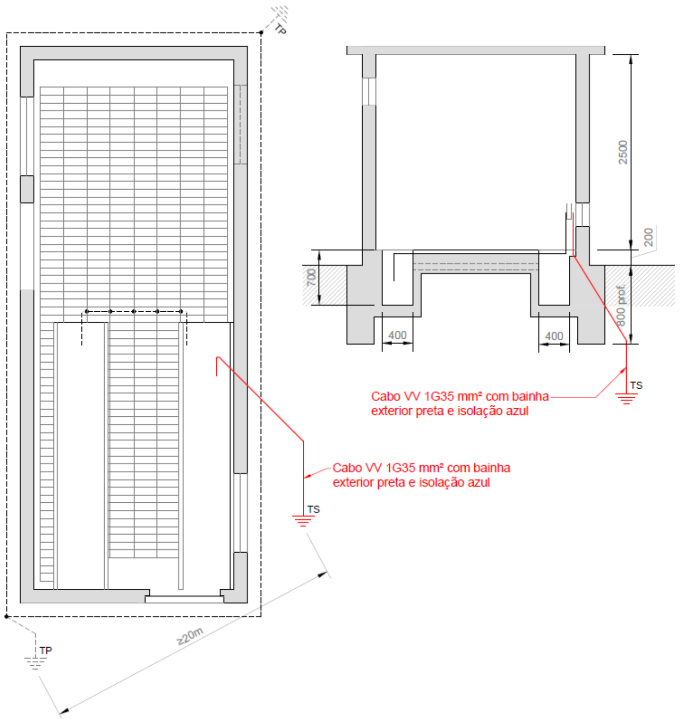
Fig. 2C – PT tipo CB • Ligação do barramento de neutro do QGBT aos elétrodos da terra de serviço
