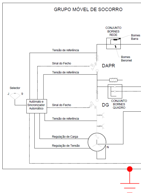
Fig. 11.2 – Grupo Móvel de Socorro (GMS) • Ligação aos eletrodos de terra
