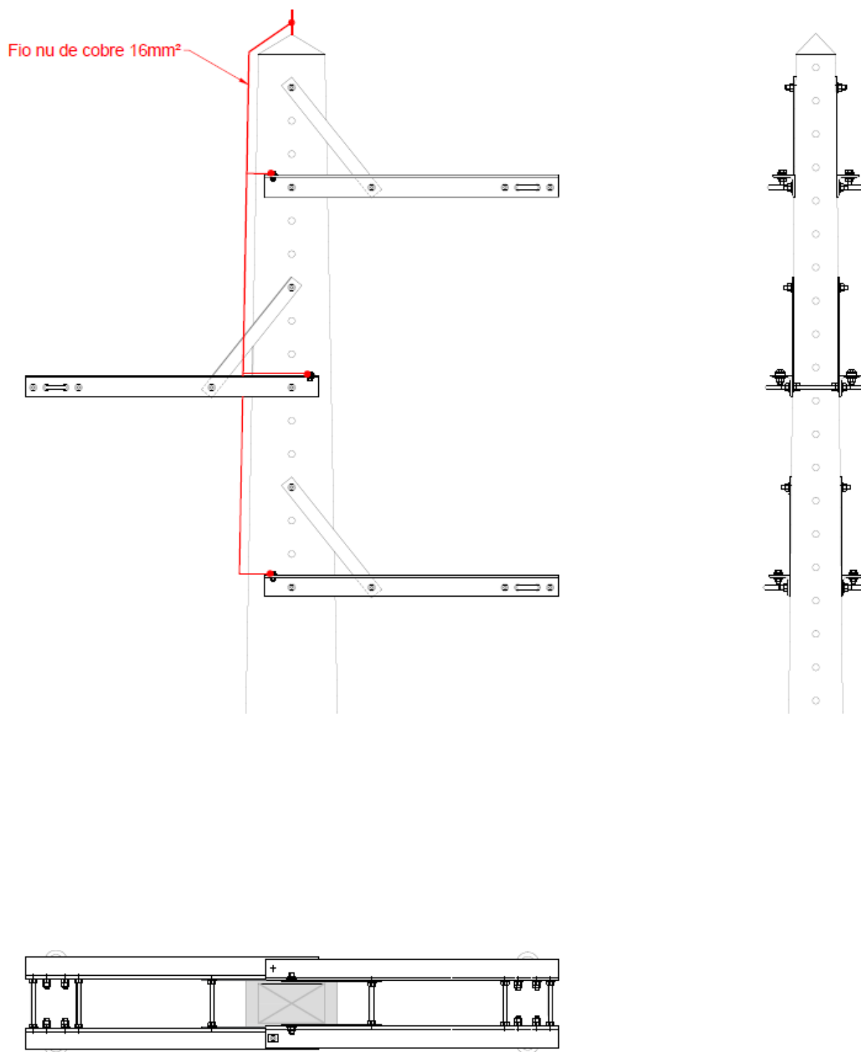
Fig. 7A – LAMT • Ligação de armação GAN à terra
