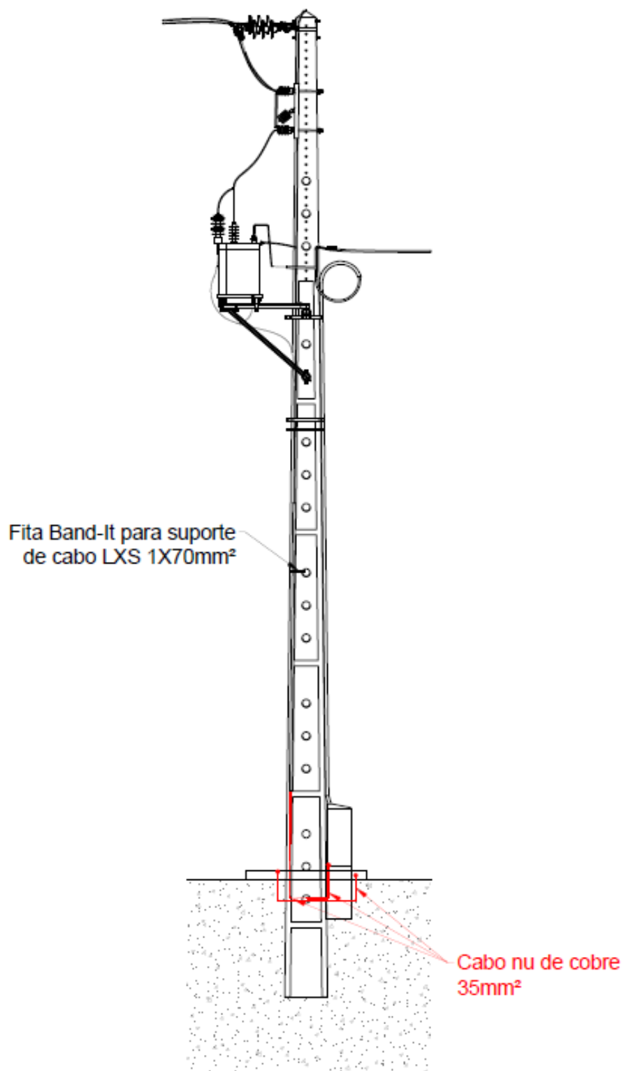
Fig. 11B – PT aéreo tipo R250 e AI • ligação das plataformas + comando do interruptor-seccionador + QGBT, à terra
