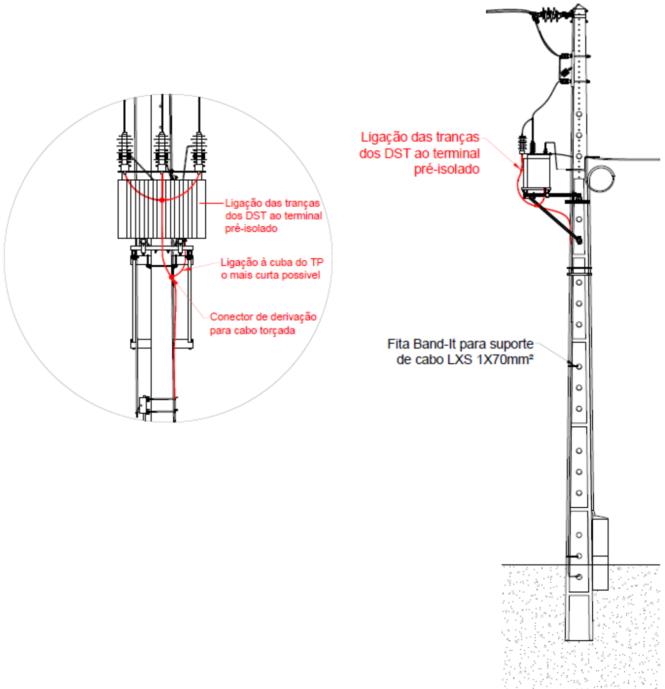
Fig. 9B – PT aéreo tipo R250 e AI • Ligação dos DST à terra e à cuba do TP
