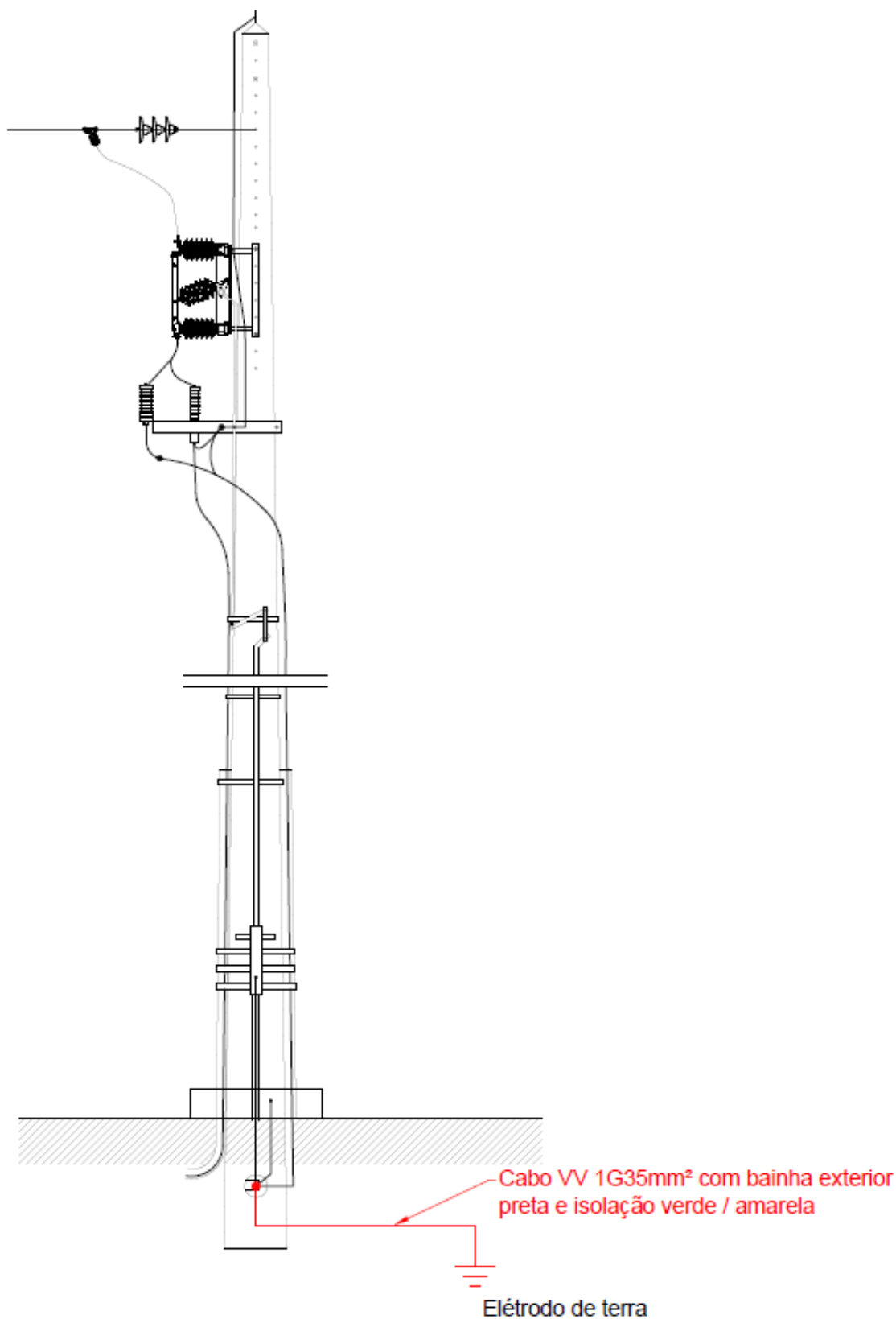
Fig. 6A – LAMT/LSMT • Ligação ao terminal inferior do poste dos elérodos de terra
