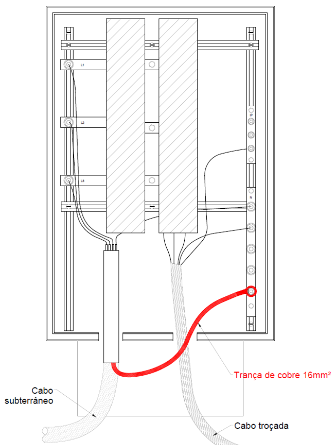
Fig. 32 - RSBT/RABT - Ligação terminação em transição aero-subterrânea
