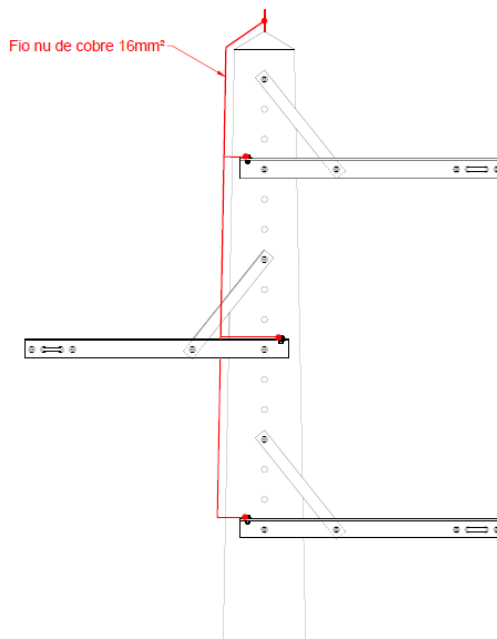
Fig. 3 – LAMT - Ligação da armação à terra
