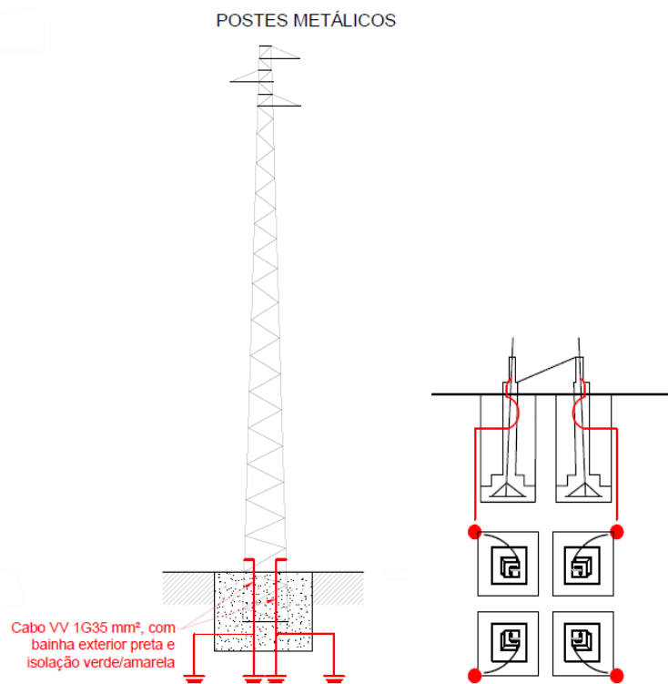
Fig. 2 – LAMT • Ligação aos eletrodos de terra
