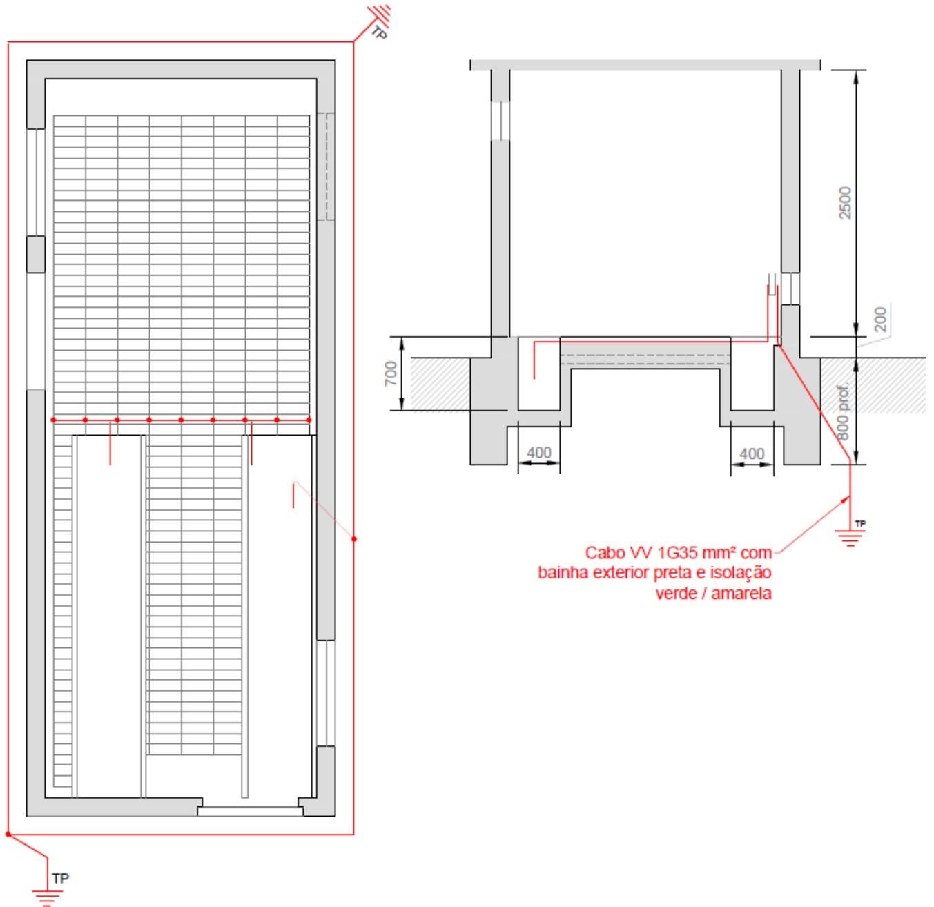
Fig. 1C – PT tipo CB • Ligação aos eletrodos de terra de proteção
