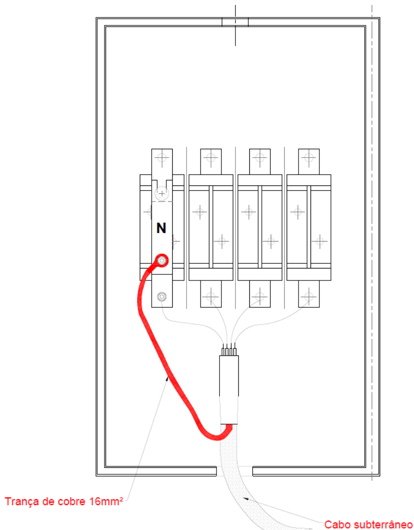
Fig. 33 - Ramais BT • Ligação das terminações à terra
