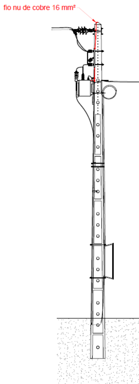
Fig. 17 - PT aéreo tipo R100•Ligação tampa e suporte TP+ armação + seccionador, à terra
