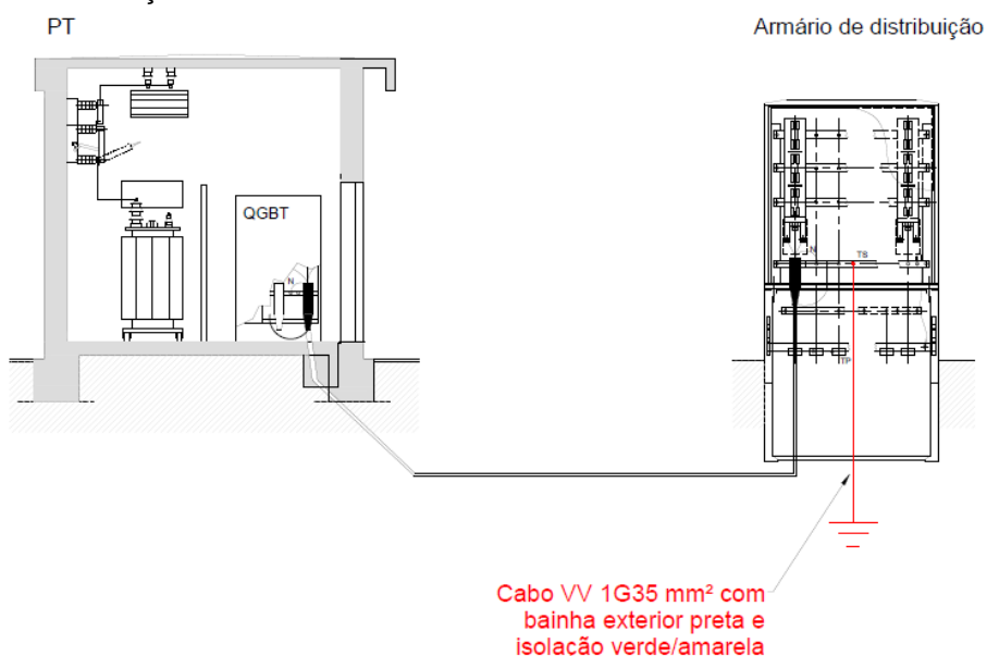
Fig. 31 – RSBT - Ligação das terminações à terra (casos particulares)
