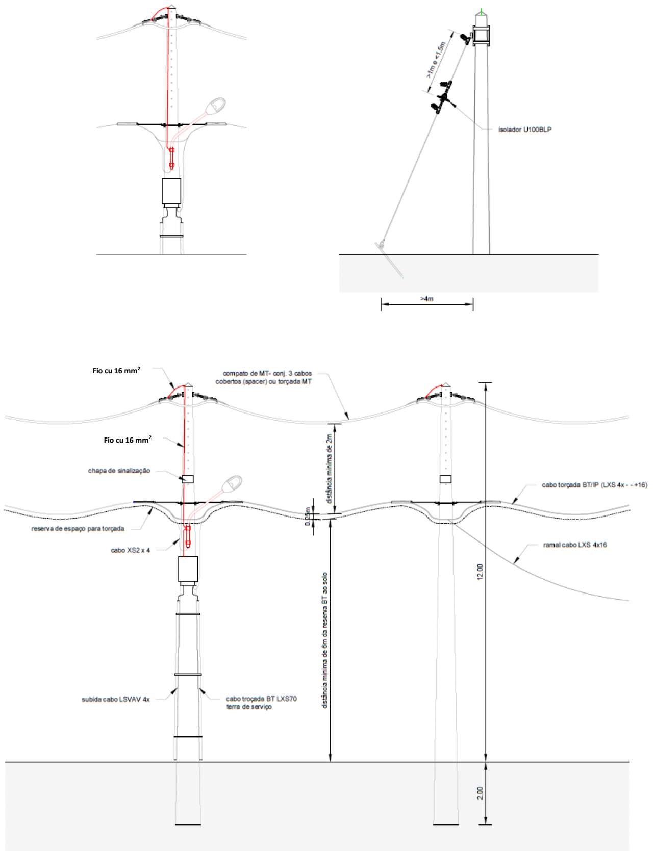
Fig. 4 – Ligação à terra do cabo tensor e dos acessórios de fixação
