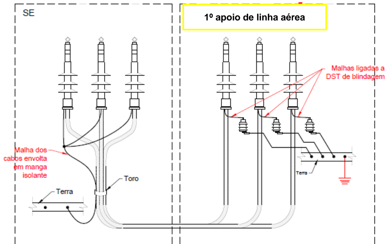
Fig. 12.2 – LSAT(MT)/LAAT(MT) • Ligação das bainhas dos cabos à terra (transição aérea-subterrânea)
