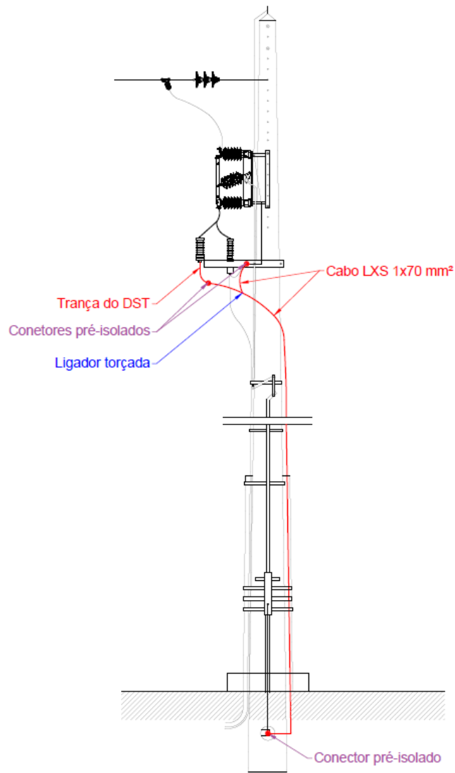
Fig. 7 – LAMT/LSMT • Ligação dos DST à terra
