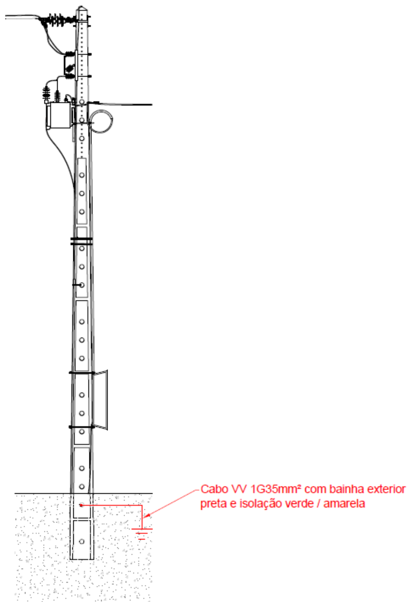
Fig. 21 - PT aéreo tipo R100 • Ligação aos elétrodos de terra
