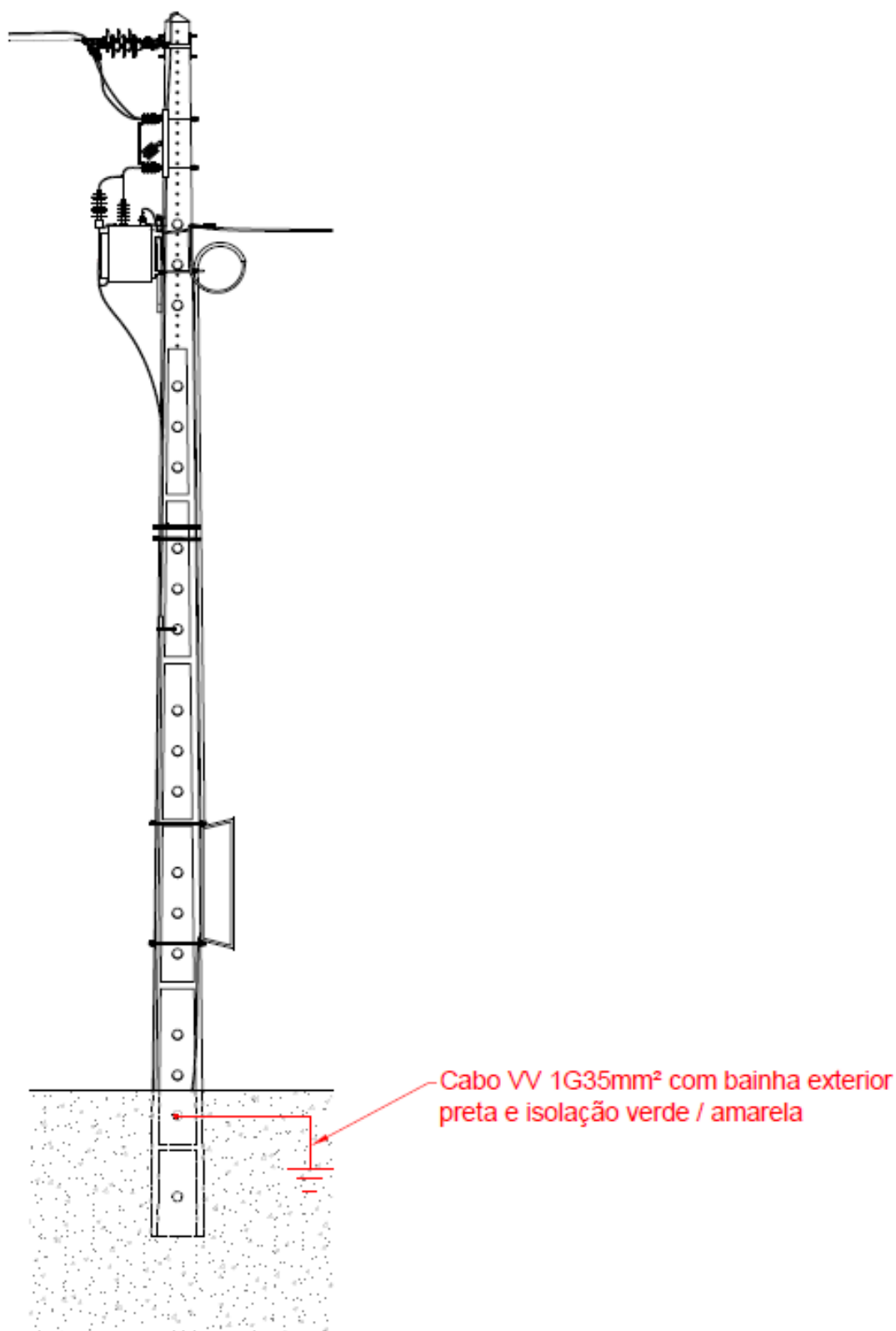
Fig. 8B – PT aéreo tipo R100 e AS • Ligação do terminal inferior do poste aos elétrodos de terra
