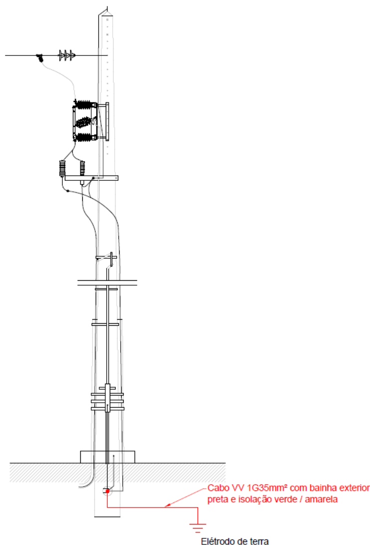
Fig. 10 – LAMT/LSMT • Ligação aos eletrodos de terra
