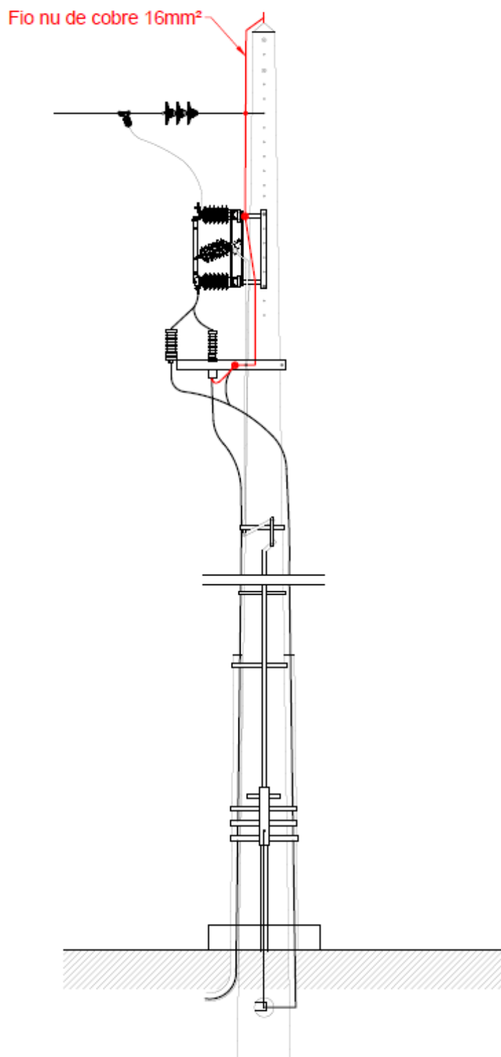
Fig. 4A – LAMT/LSMT • Ligação armação + armação de fim cabo + seccionador à terra
