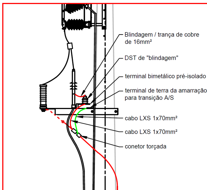
Fig. 12.3 – Ligação da blindagem à terra de proteção por intermédio de DST de "blindagem"
