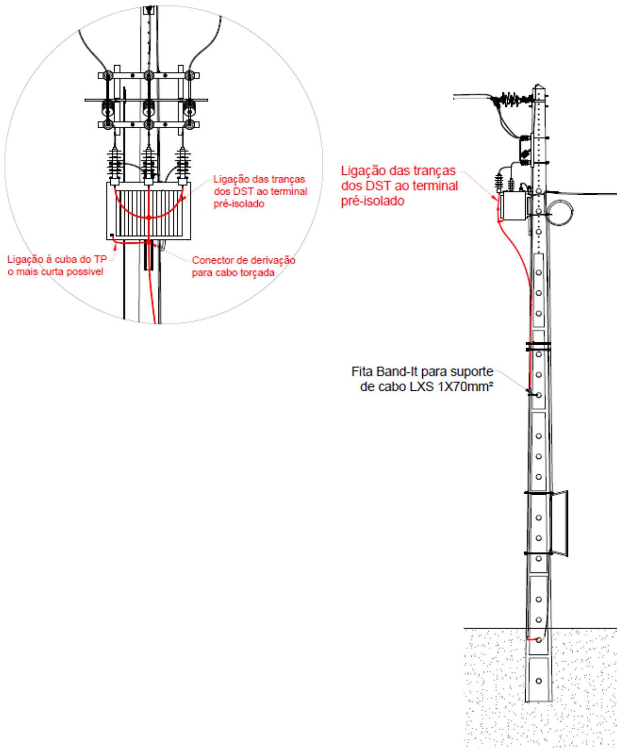
Fig. 5B – PT aéreo tipo R100 e AS • Ligação dos DST à terra e à cuba do TP
