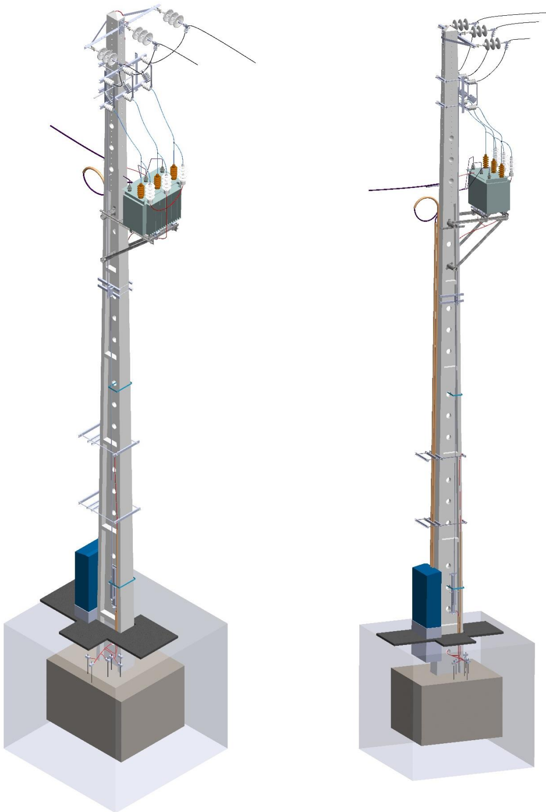
Fig. 15B - PT aéreo tipo R250 e AI • representação 3D.
