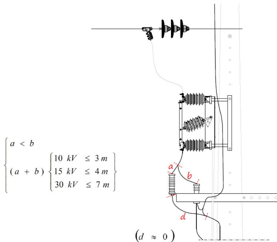
Fig. 6B – Ligação dos DST (distâncias a observar aos equipamentos a proteger)
