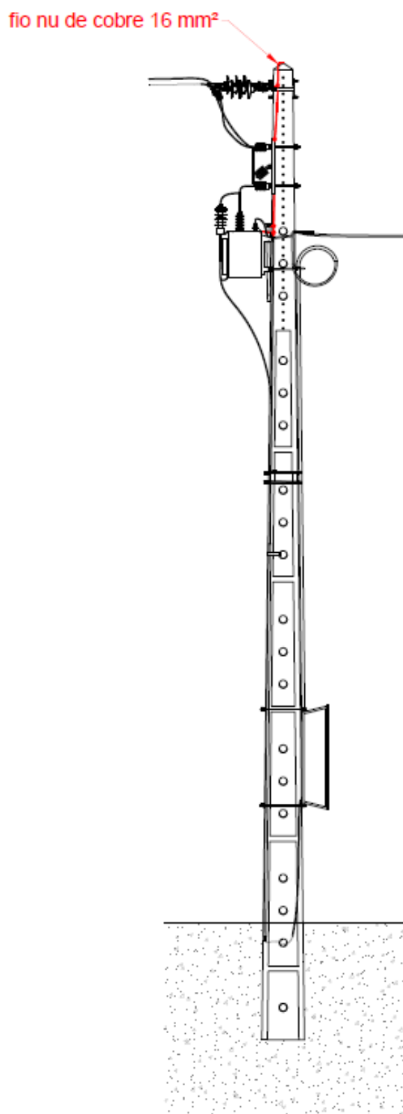
Fig. 6B – PT aéreo tipo R100 e AS • Ligação da armação de suspensão e tampa de TP + seccionador + HPT4, à terra
