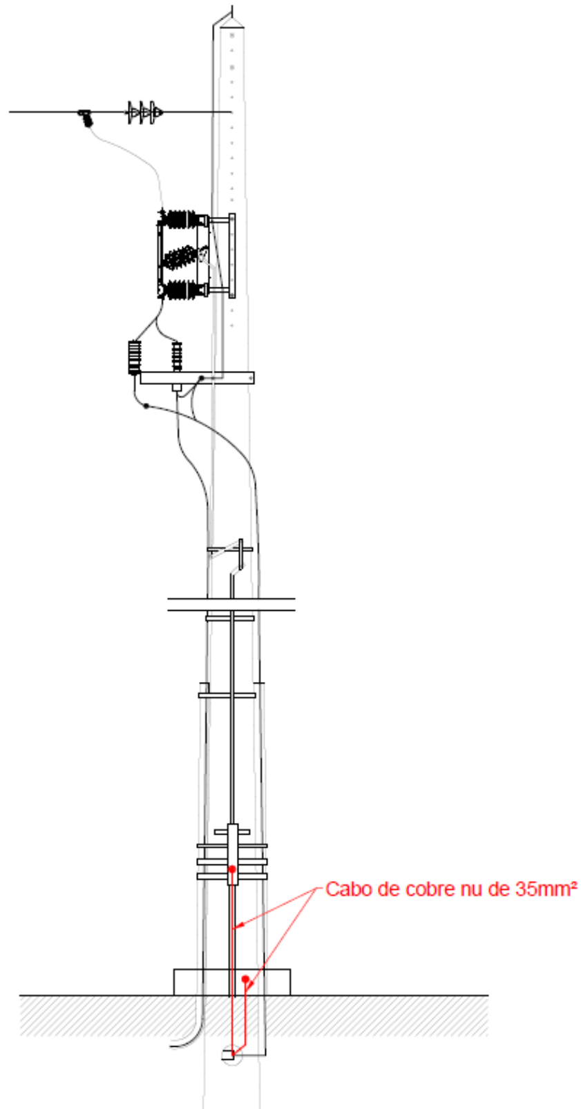
Fig. 5A – LAMT/LSMT • Ligação das plataformas + comando seccionador à terra
