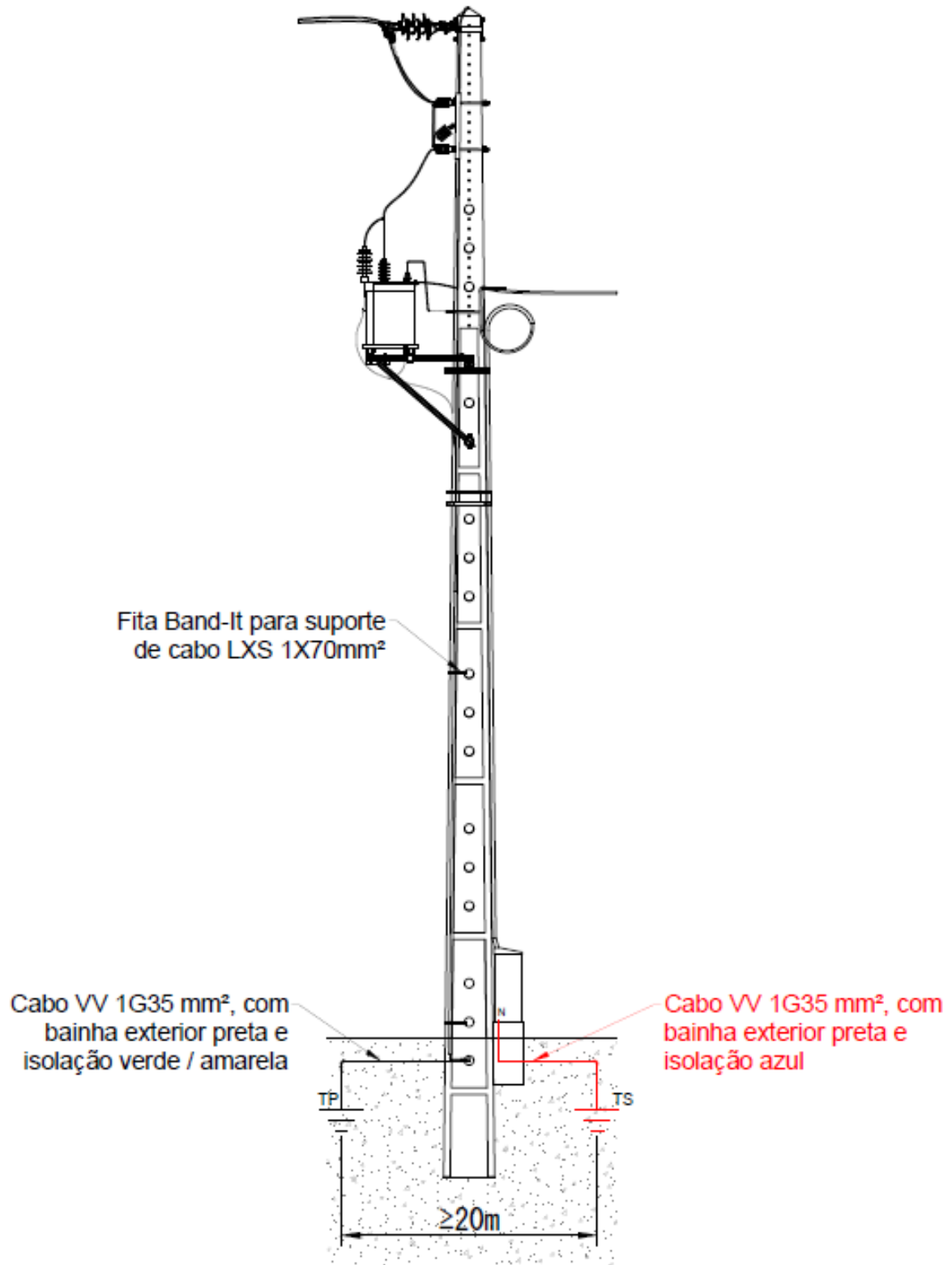
Fig. 13B - PT aéreo tipo R250 e AI • Ligação barramento de neutro do QGBT aos elétrodos de terra de serviço.
