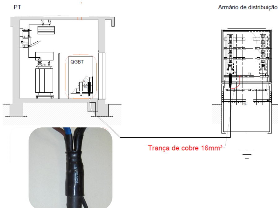
Fig. 30.1 - RSBT • Ligação das terminações à terra
