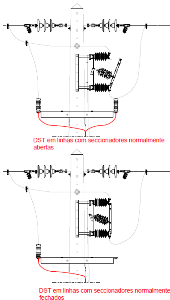
Fig. 6 – LAMT – DST em postes com seccionador
