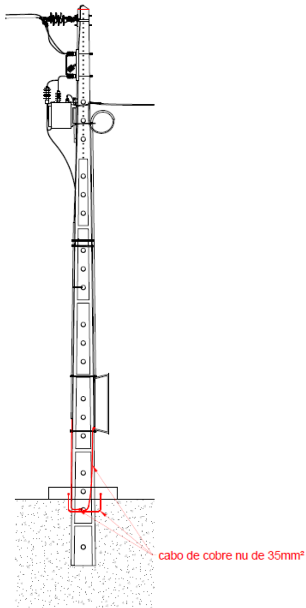
Fig. 19 - PT aéreo tipo R100•Ligação do comando seccionador + plataformas + QGBT à terra
