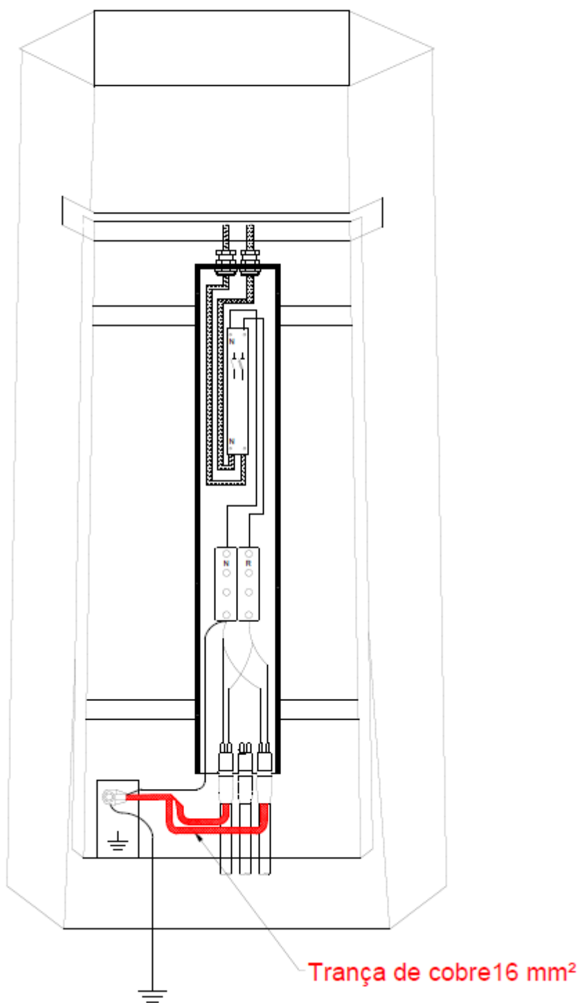
Fig. 3F – RSIP • Ligação das terminações dos cabos subterrâneos ao terminal do fuste da coluna
