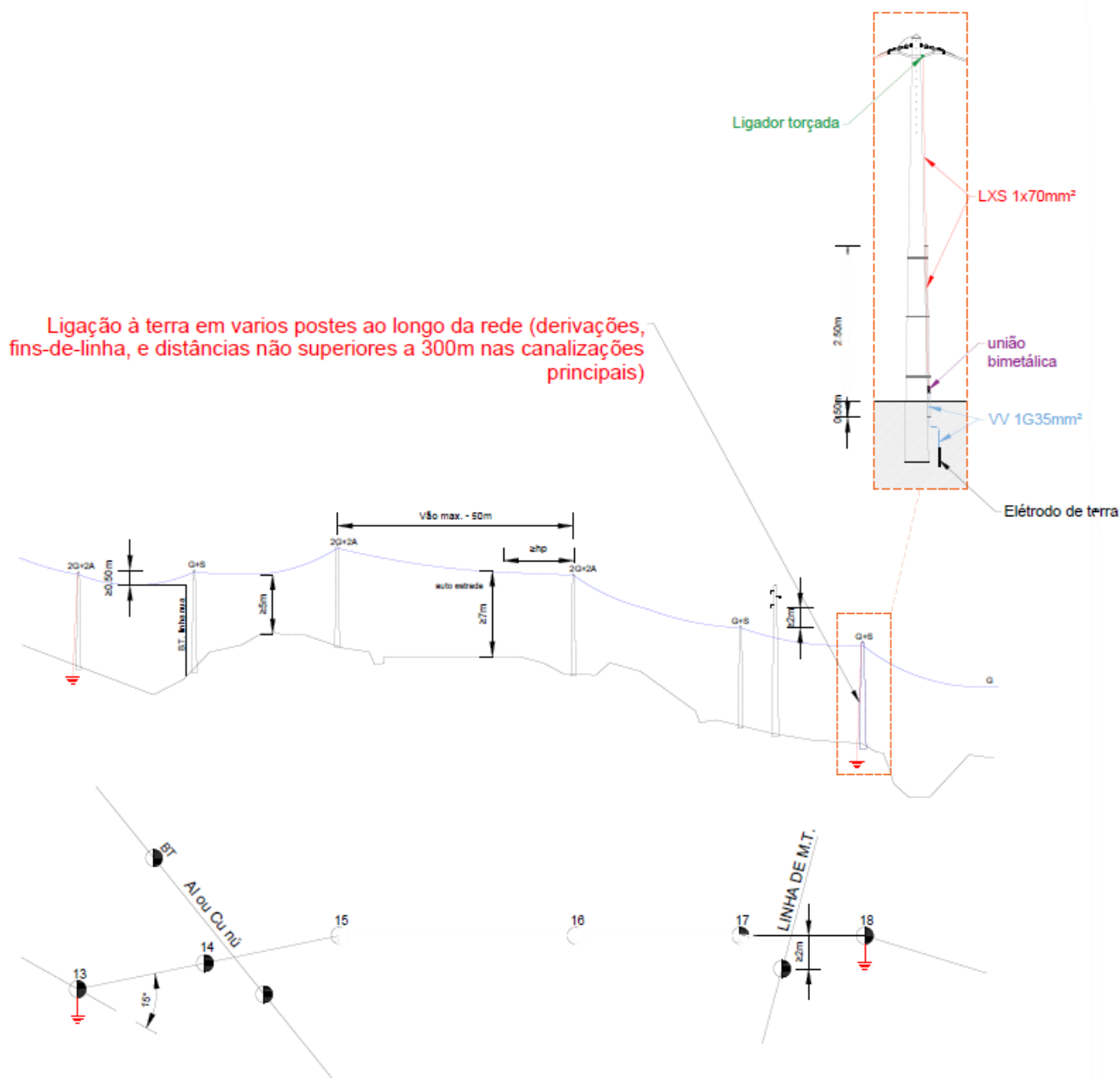
Fig. 28 - RABT • Ligação do neutro à terra
