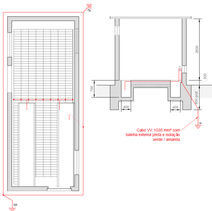
Fig. 25 – PT tipo CB • Ligação aos eletrodos de terra de proteção
