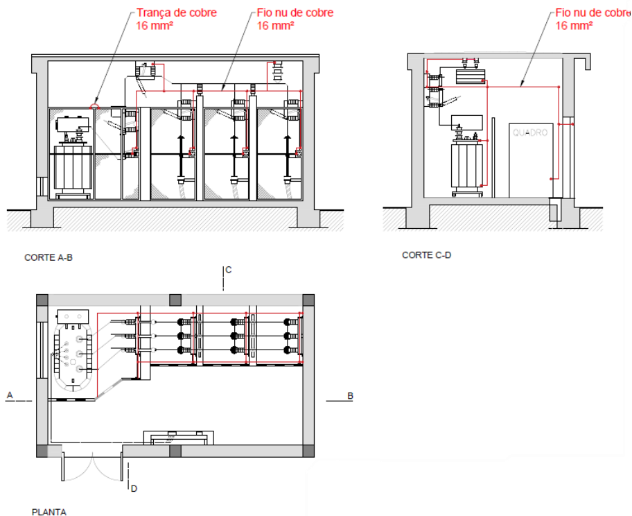
Fig. 24 – PT tipo CB • Ligação das partes metálicas à terra de proteção
