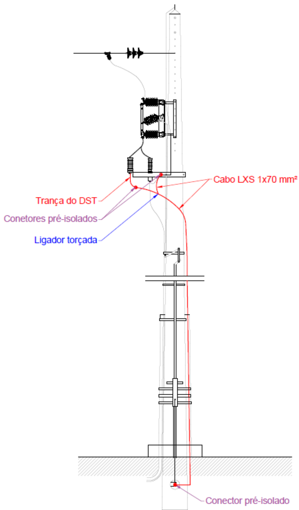
Fig. 3A – LAMT/LSMT • Ligação dos DST à terra
