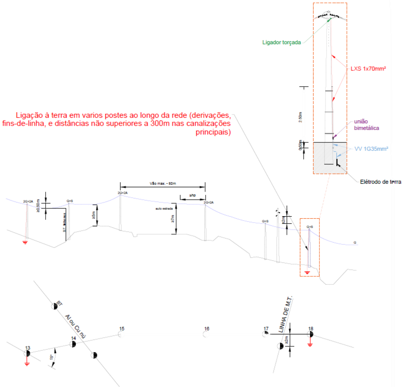
Fig. 1D – RABT • Ligação do neutro à terra
