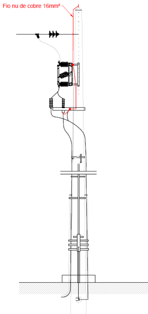
Fig. 8 – LAMI/LSMT • Ligação armação.+ caixas + seccionador à terra
