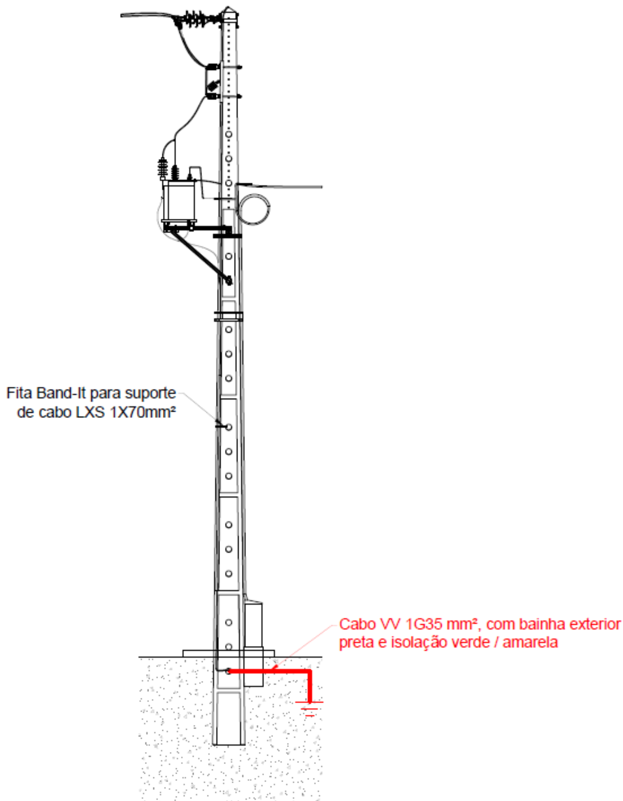
Fig. 12B – PT aéreo tipo R250 e AI • Ligação do terminal inferior do poste aos elétrodos de terra de proteção
