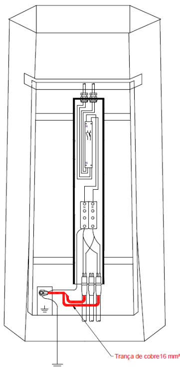
Fig. 36 – RSIP - Ligação das terminações dos cabos à terra
