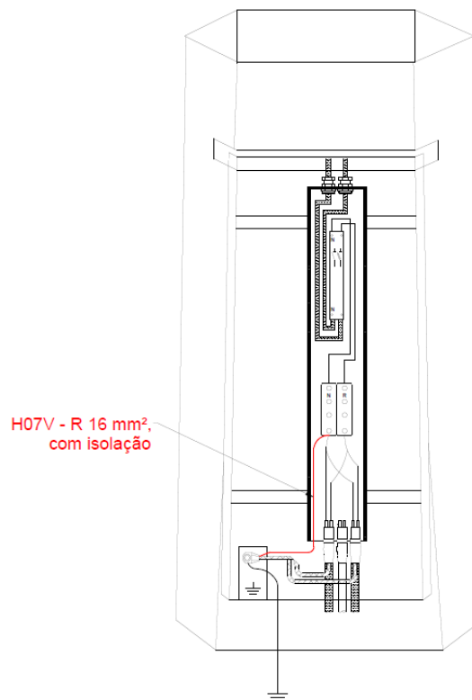
Fig. 35 – RSIP - Ligação do quadro de IP à terra do poste
