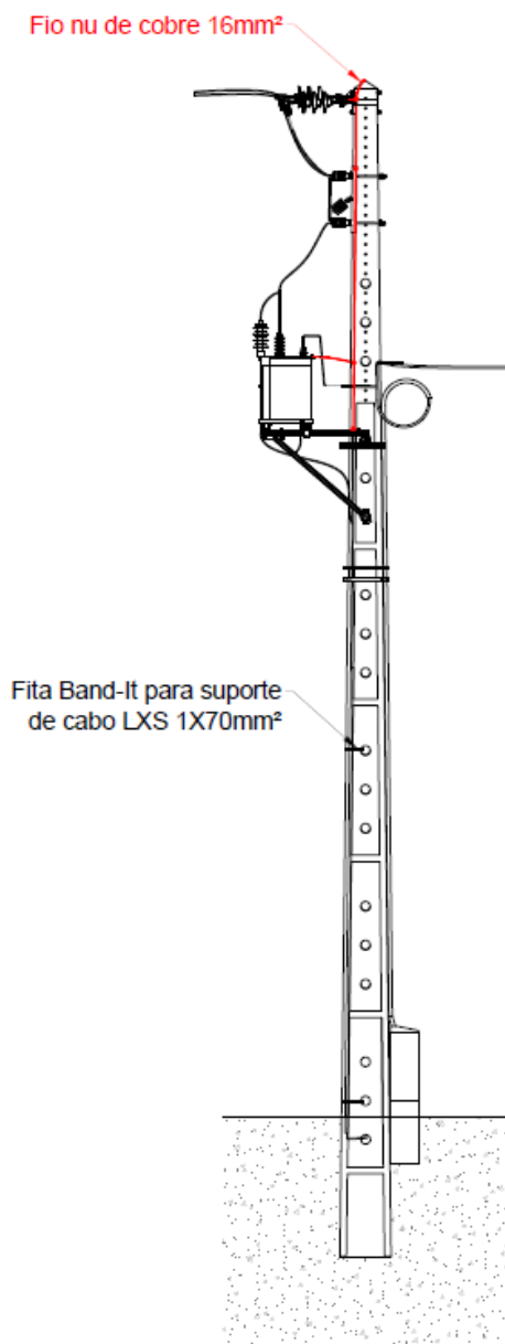
Fig. 18 - PT aéreo tipo R250 • Ligação terminal superior, tampa TP + interruptor-seccionador + armação à terra
