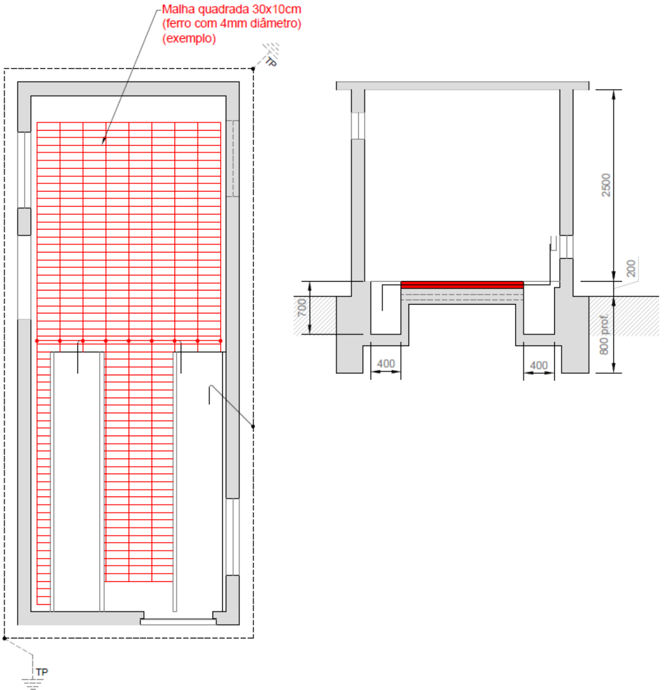
Fig. 3C – PT tipo CB • Ligação da malha equipotencial à terra de proteção
