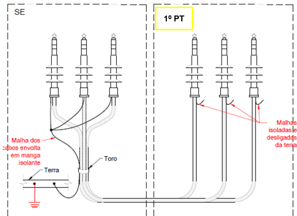
Fig. 12.1 – LAAT(MT)/LSAT(MT) • Ligação das bainhas dos cabos à terra (PT alimentado diretamente por SE)
