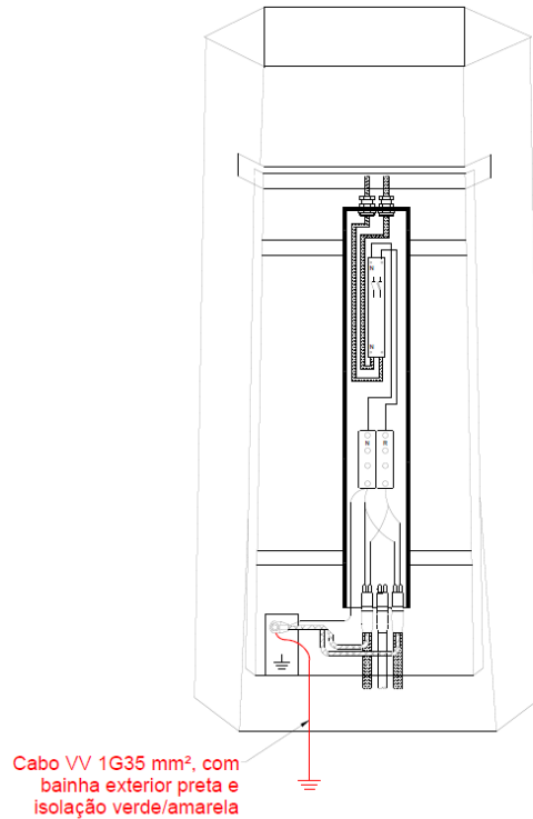
Fig. 34 – RSIP - Ligação terminal terra do poste à terra
