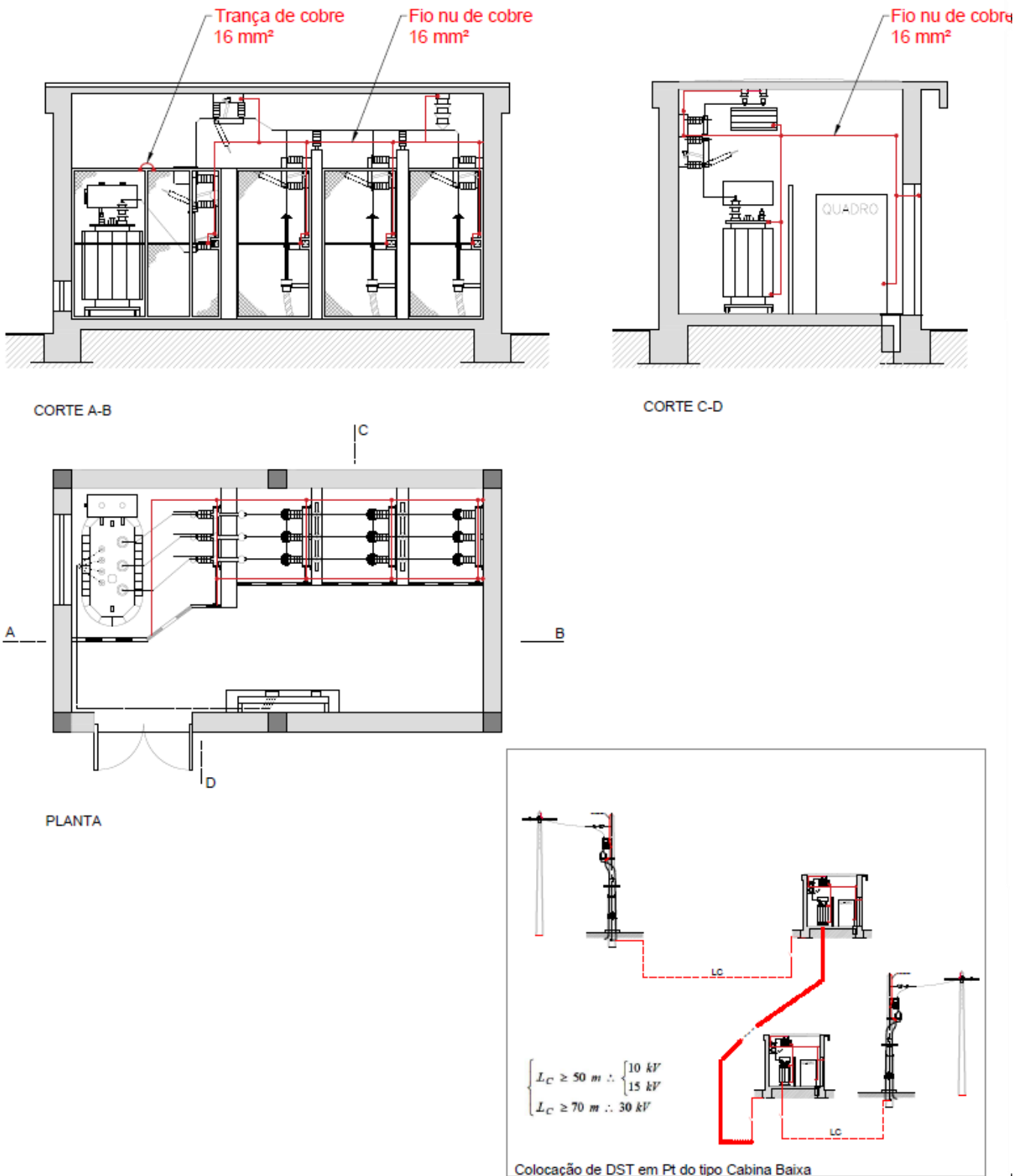
Fig. 4C – PT tipo CB • Ligação das massas metálicas à terra de proteção
