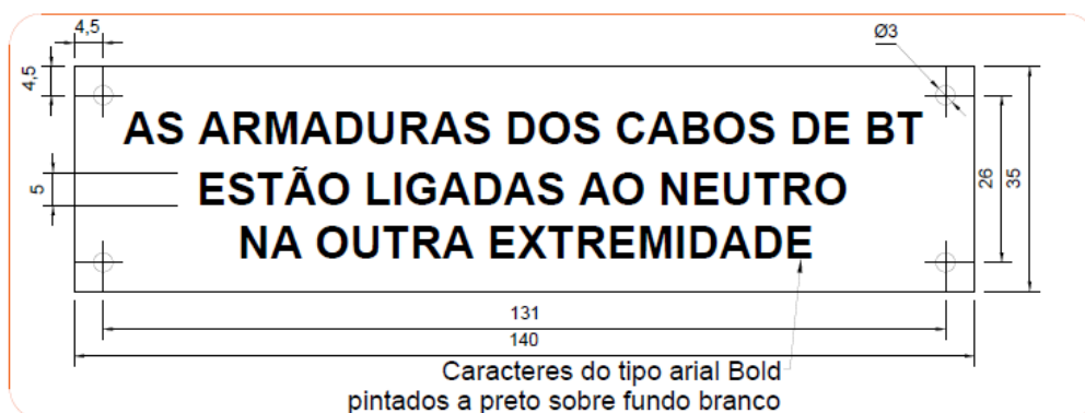
Fig. 30.2 – PT tipo CB • Aviso com a indicação do local de ligação das armaduras ao neutro
