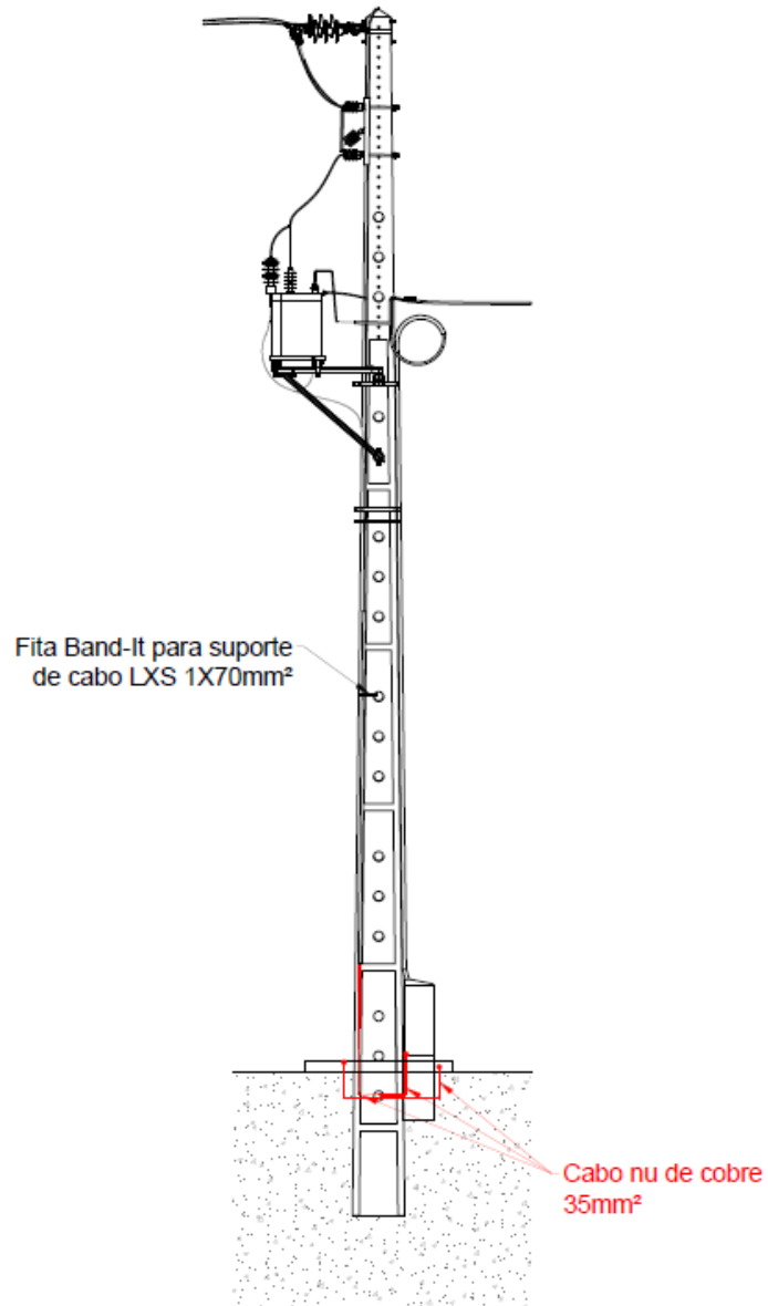
Fig. 20 - PT aéreo tipo R250 • Ligação comando interruptor-seccionador + plataformas + QGBT, à terra
