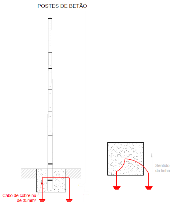
Fig. 1 – LAMT • Ligação aos elétrodos de terra
