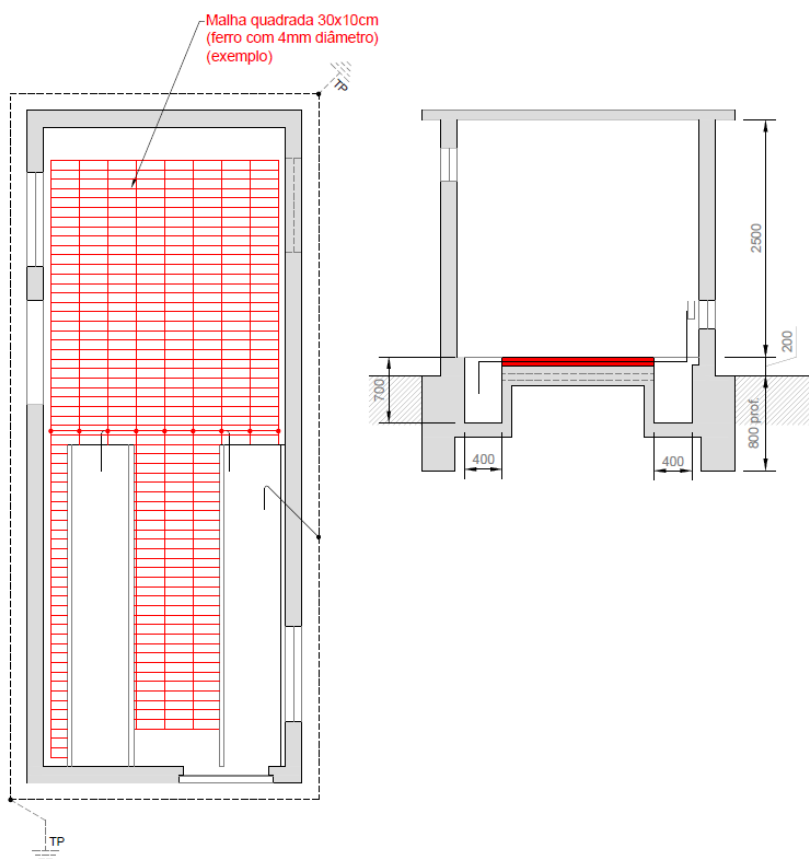
Fig. 26 – PT tipo CB • Ligação da malha equipotencial à terra
