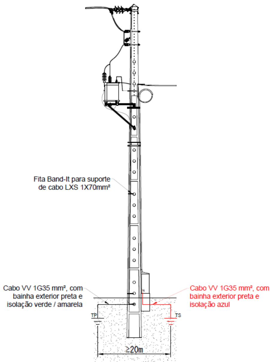
Fig. 22 - PT aéreo tipo R250 • Ligação do neutro à terra
