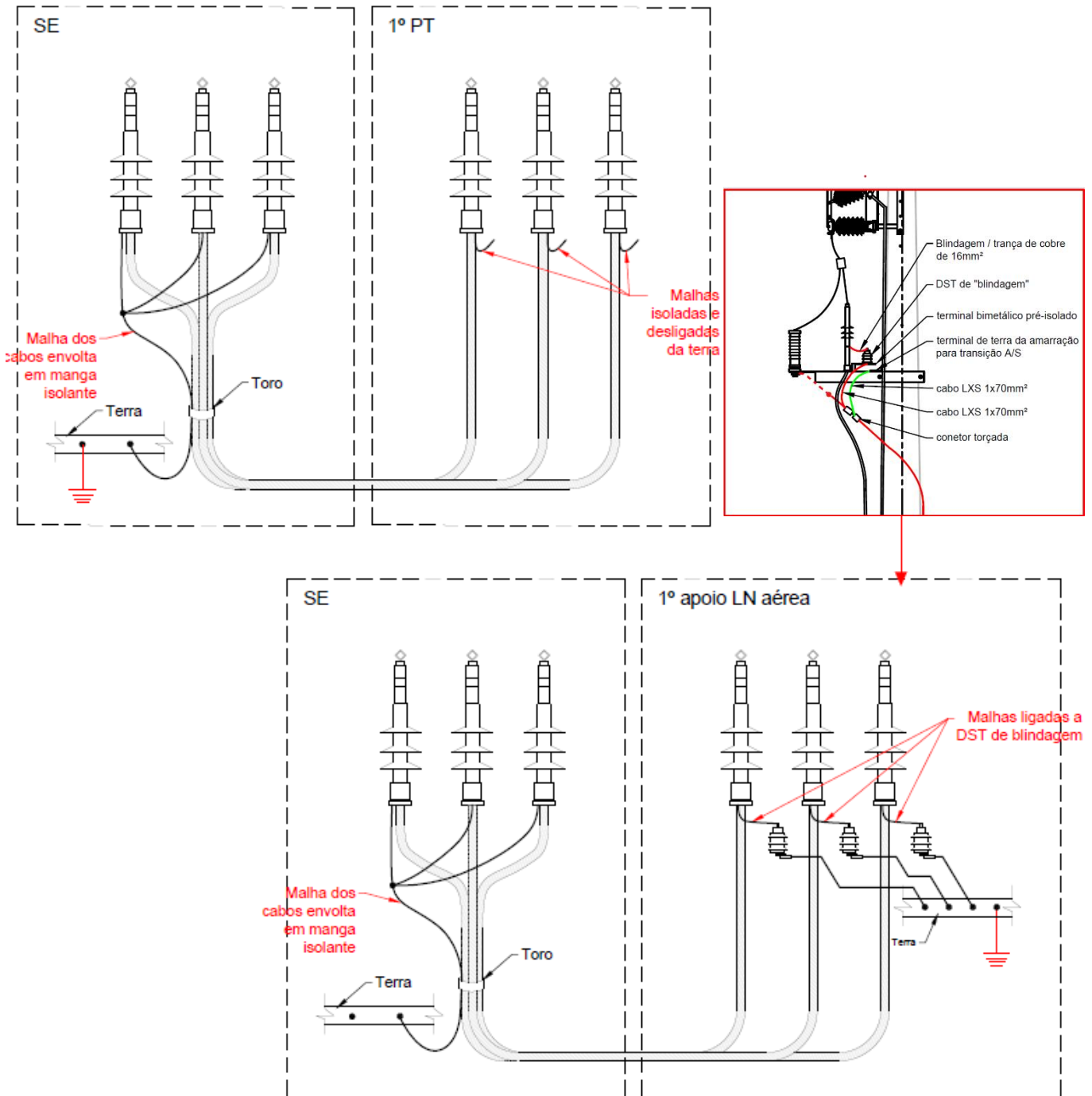
Fig. 9A – LAAT(MT)/LSAT(MT) • Ligação das terminações dos cabos subterrâneos em SE AT/MT, à terra
