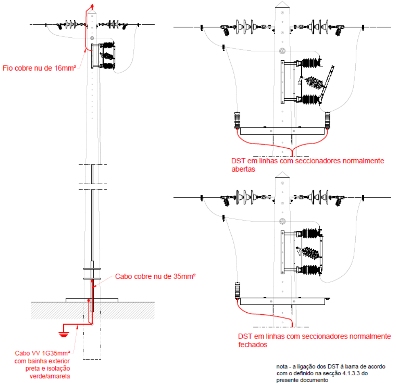
Fig. 2A – LAMT Ligação à terra de poste com seccionador
